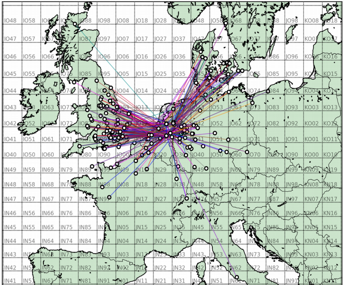
QSO's vanuit Nederland op 144 MHz
