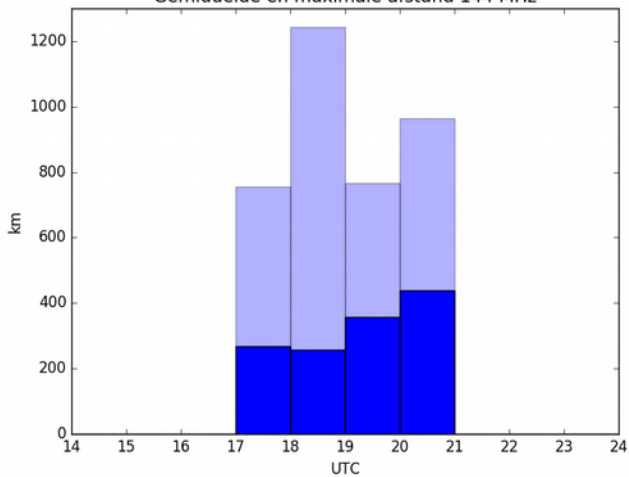
Gemiddelde en maximale afstand 144 MHz
